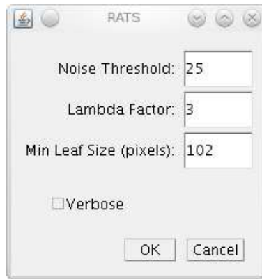
Rysunek 6. Okno algorytmu segmentacji podziału obszaru algorytmem RATS.
