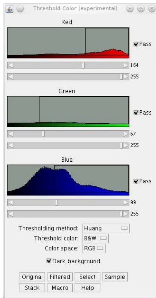
Rysunek 3. Okno Threshold Color dla przestrzeni kolorów RGB.
