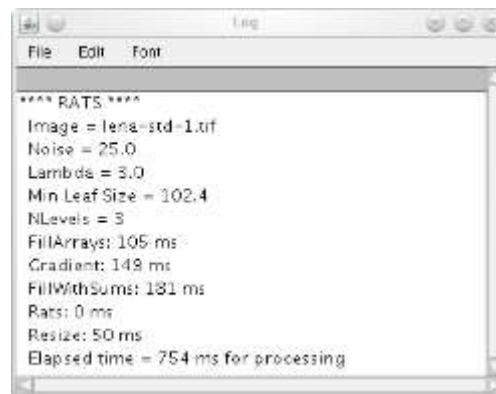
Rysunek 7. Log danych dotyczących podziału przeprowadzonego algorytmem RATS.
